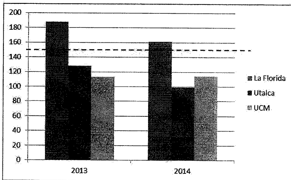
Figura 6. Percentil 98 de las concentraciones diarias de MP10 Periodo de evaluación: 21-03-2013 a 30-11-2014. Estación La Florida comenzó a medir a fines de marzo de 2013 y hay pérdida de datos de MP10 en junio, julio y agosto de 2013. Datos referenciales.
