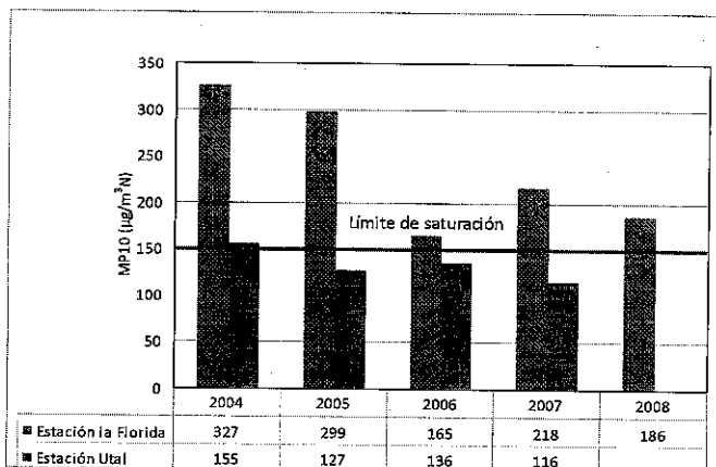
Figura 4. Percentil 98 de concentración diaria de MP10 – Talca
