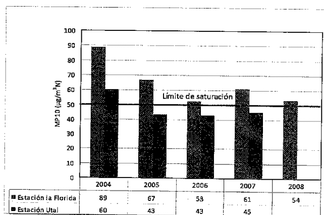
Figura 5. Concentración promedio anual de MP10 – Talca
